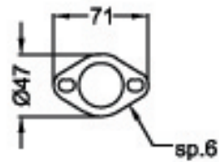
Vista da "B" Flangia "43B"
