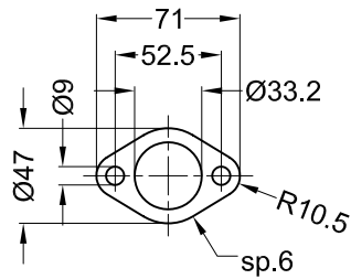
Flangia "43A"
